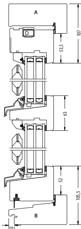
Vertikalsnitt
