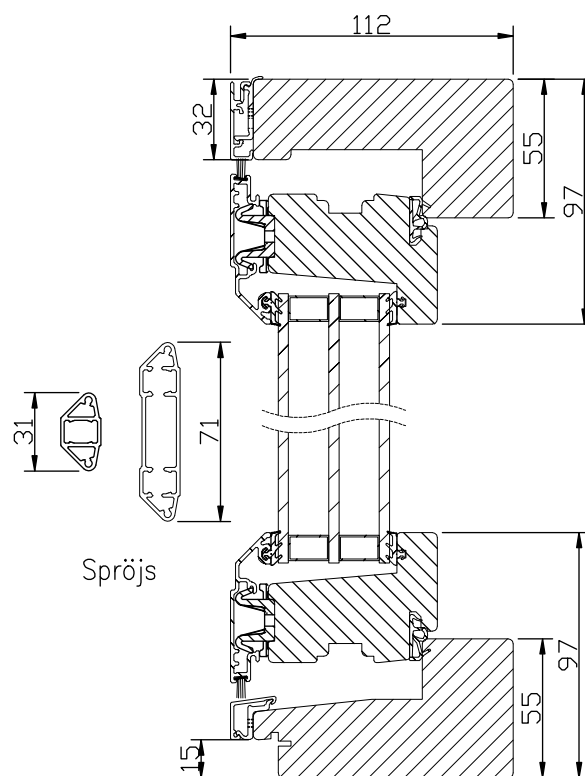
Vertikalsnitt
