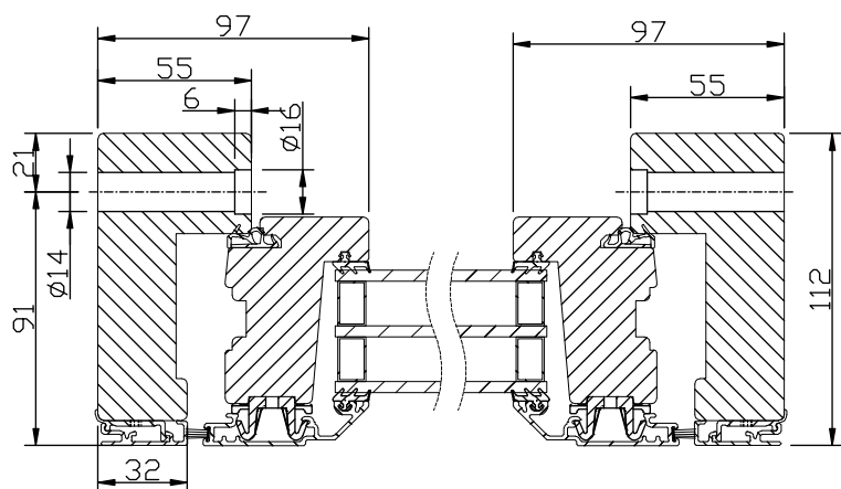
Horizontalsnitt bågpost
