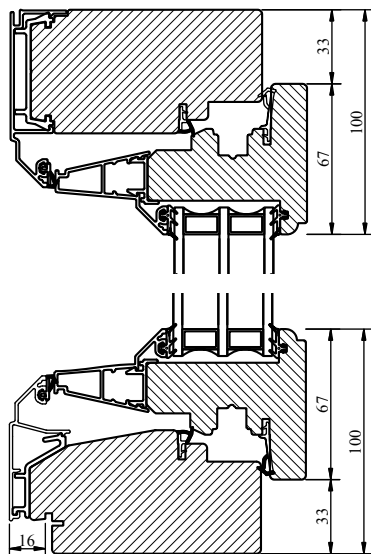
Vertikalsnitt
