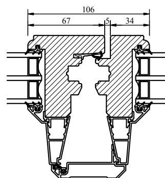
Horizontalsnitt mötesbåge
