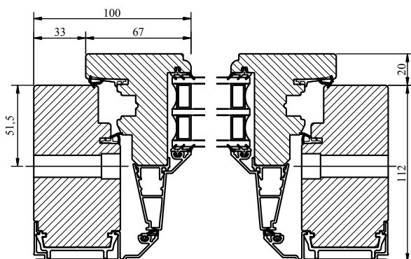
Horizontalsnitt
