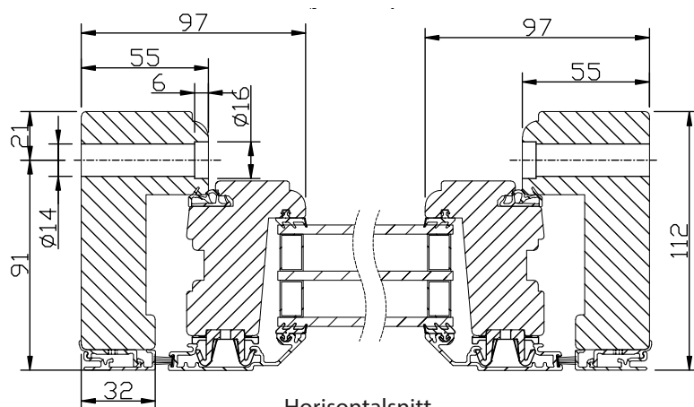
Horizontalsnitt
