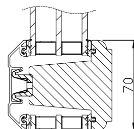
Vertikalsnitt bågpost
