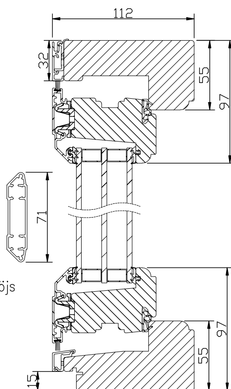
Vertikalsnitt
